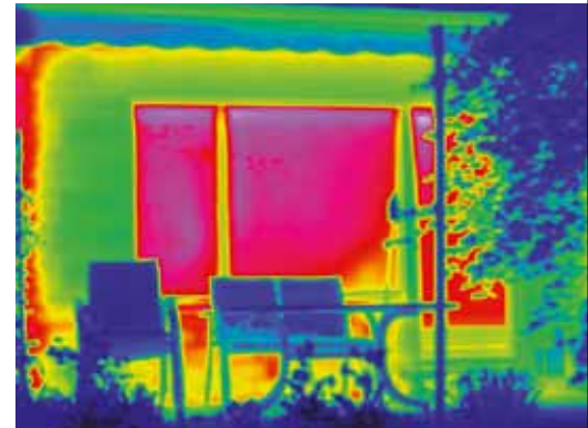
Infraroodopnames – thermografieën – tonen duidelijk aan waar een huis ongecontroleerd energie verliest. Rood betekent warmte en zodoende energieverlies.
